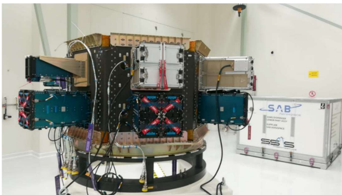
Assemblage des différents nano-satellites tels qu’ils seront dans la fusée. AMICal Sat, dans son POD, en haut à gauche de la photo ©SAB Aérospace
